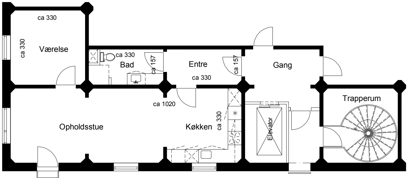
Plantegning
