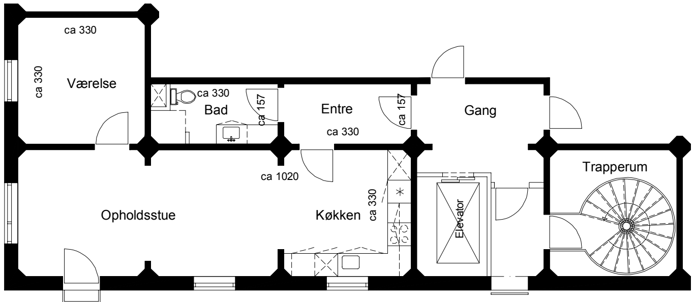
Plantegning
