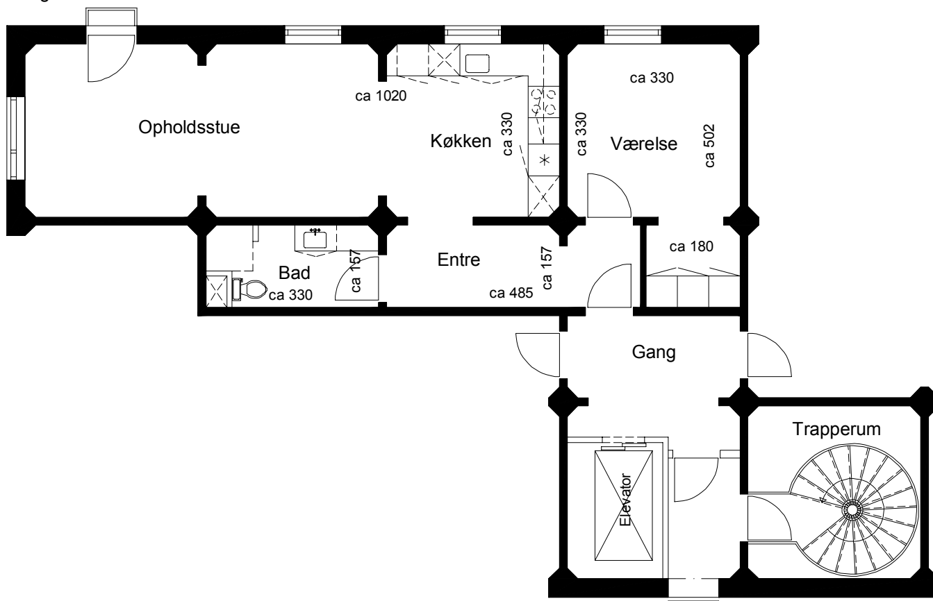
Plantegning
