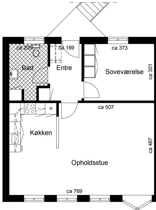
Plantegning
