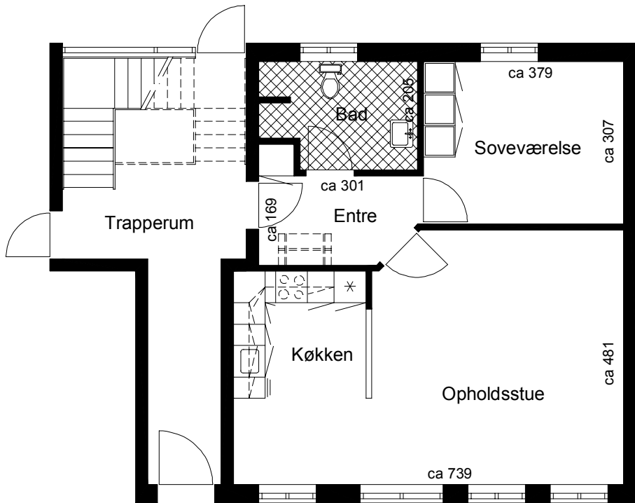
Plantegning
