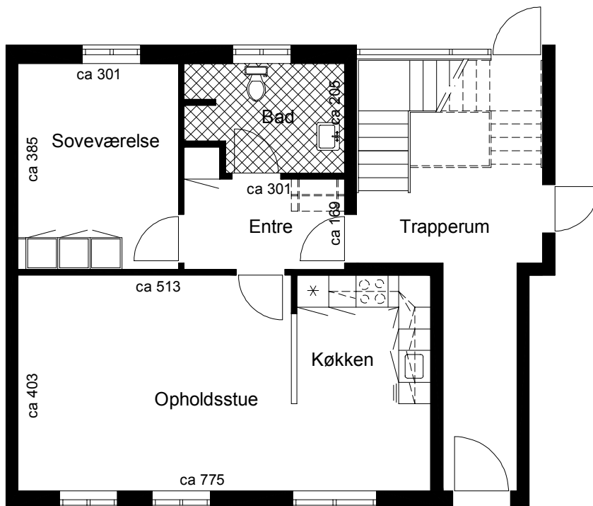
Plantegning
