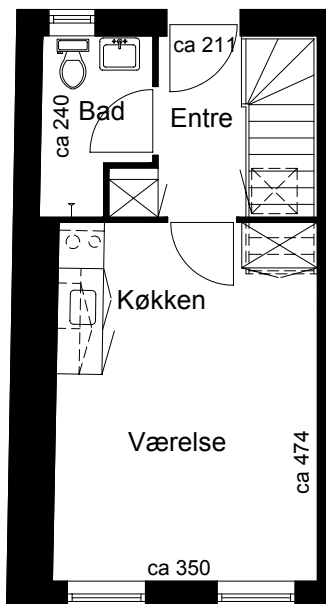
Plantegning
