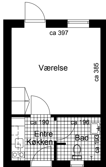
Plantegning
