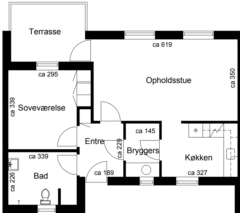
Plantegning
