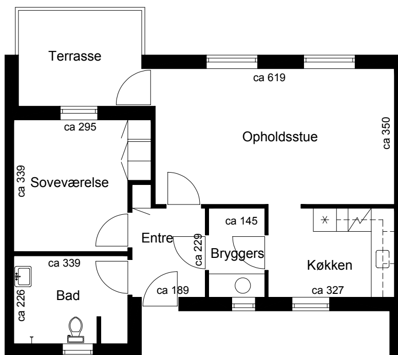
Plantegning
