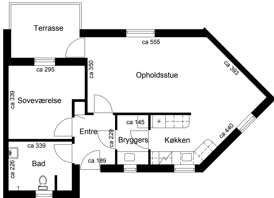
Plantegning
