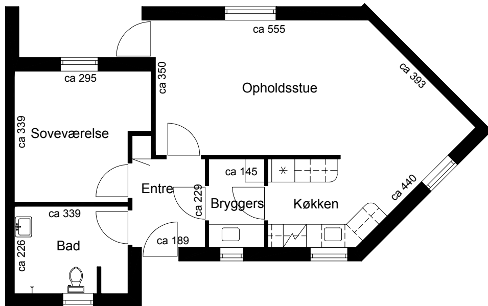
Plantegning
