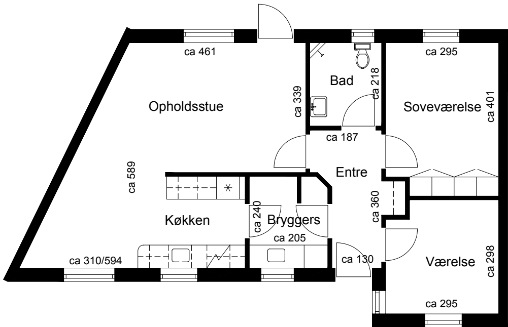
Plantegning
