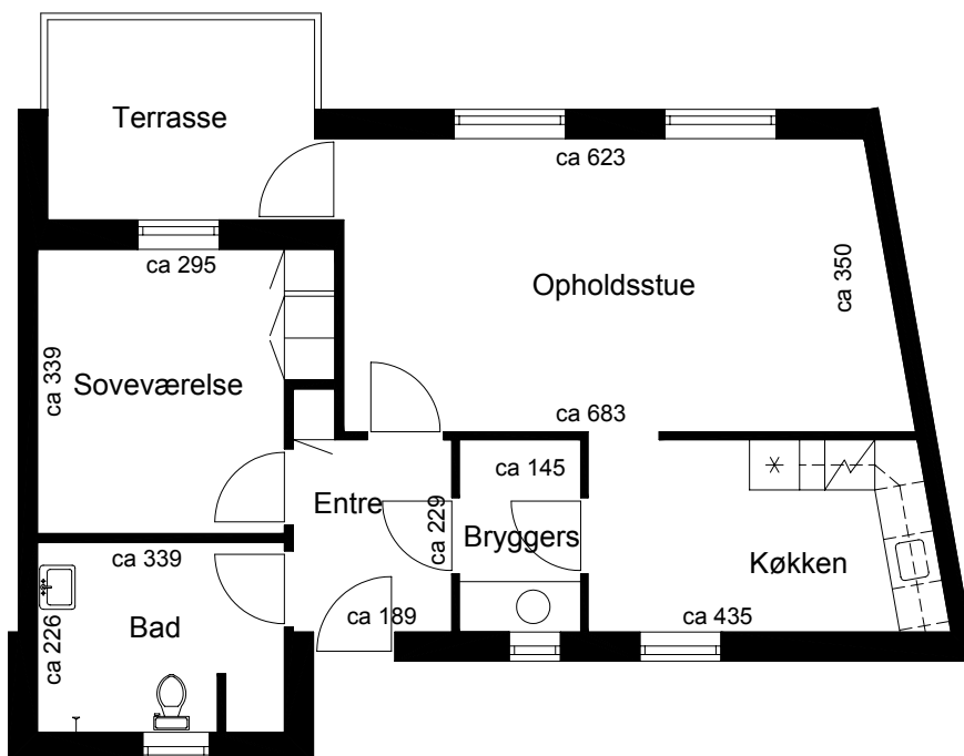
Plantegning
