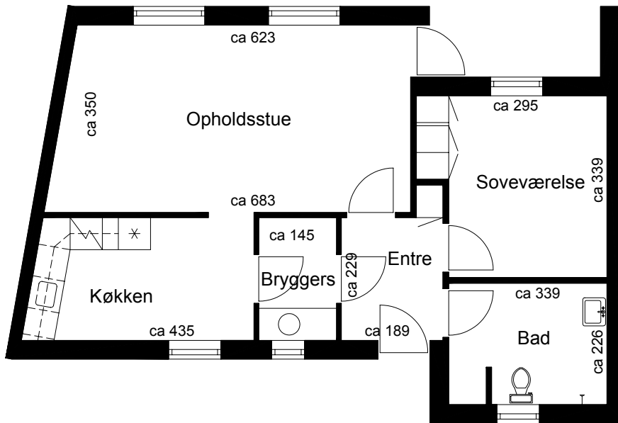
Plantegning
