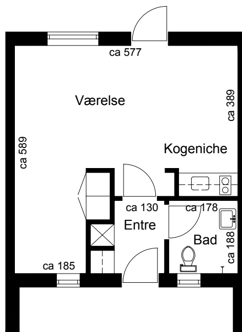
Plantegning
