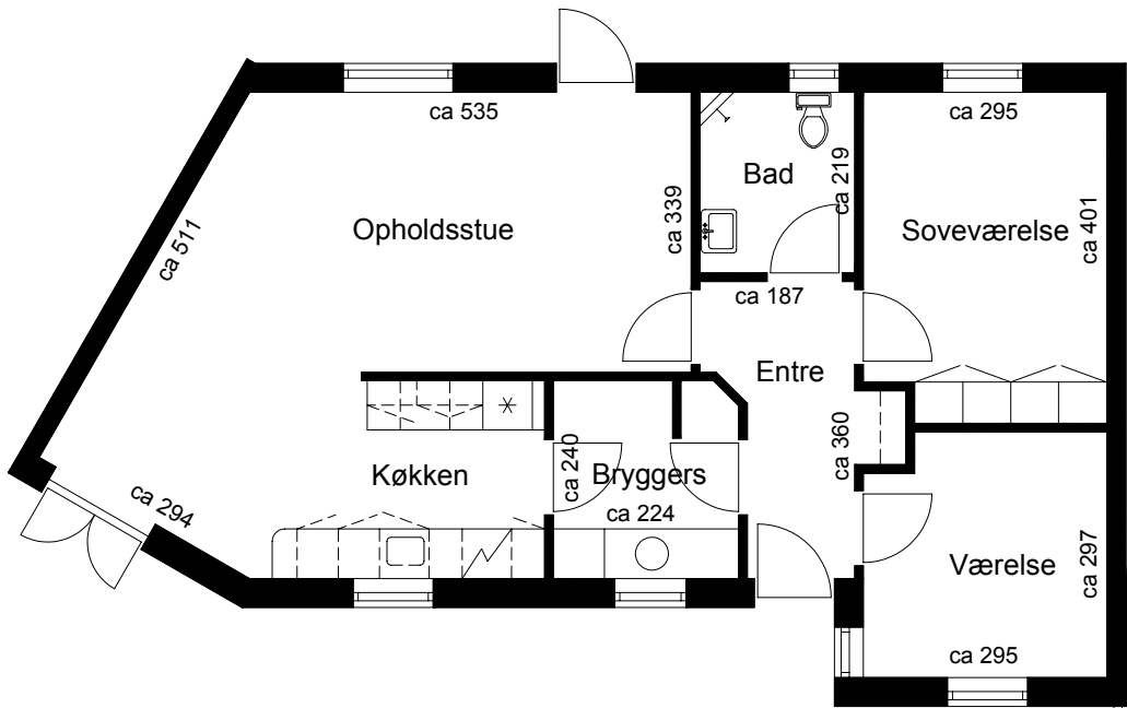
Plantegning
