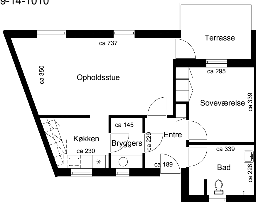
Plantegning
