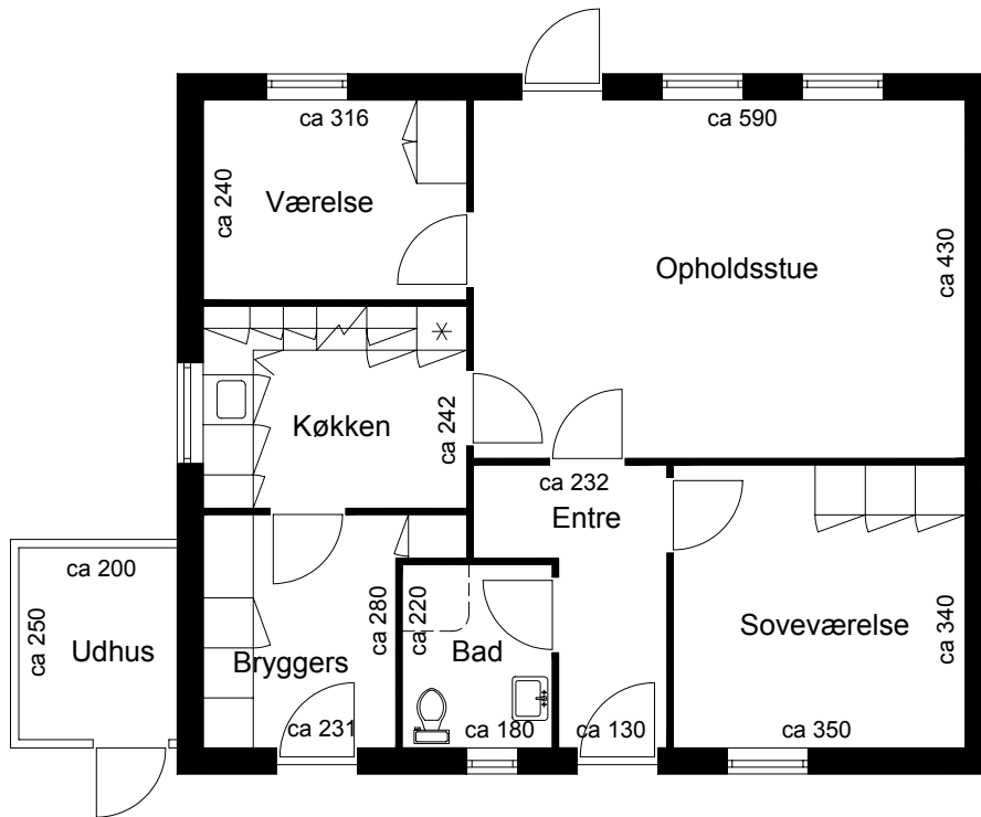
Plantegning
