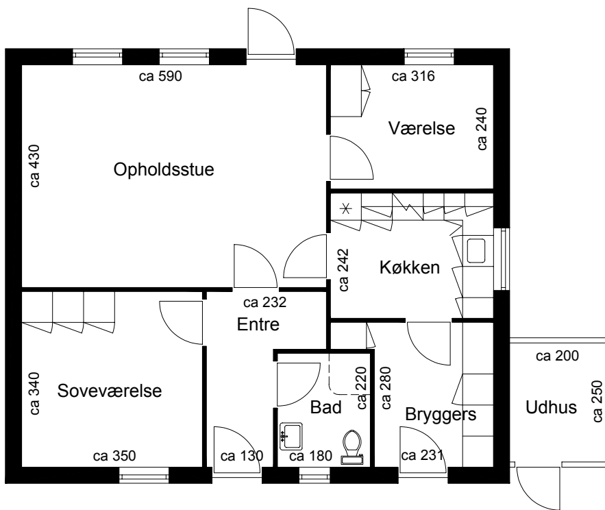
Plantegning
