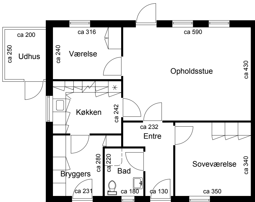
Plantegning
