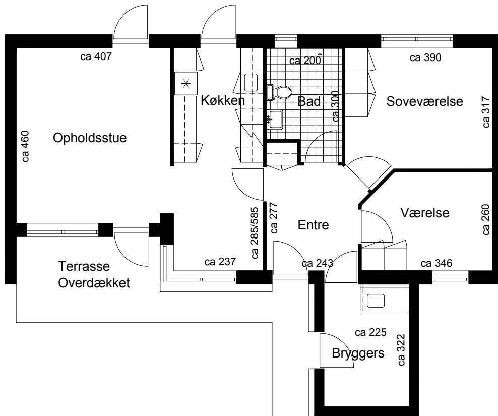
Plantegning
