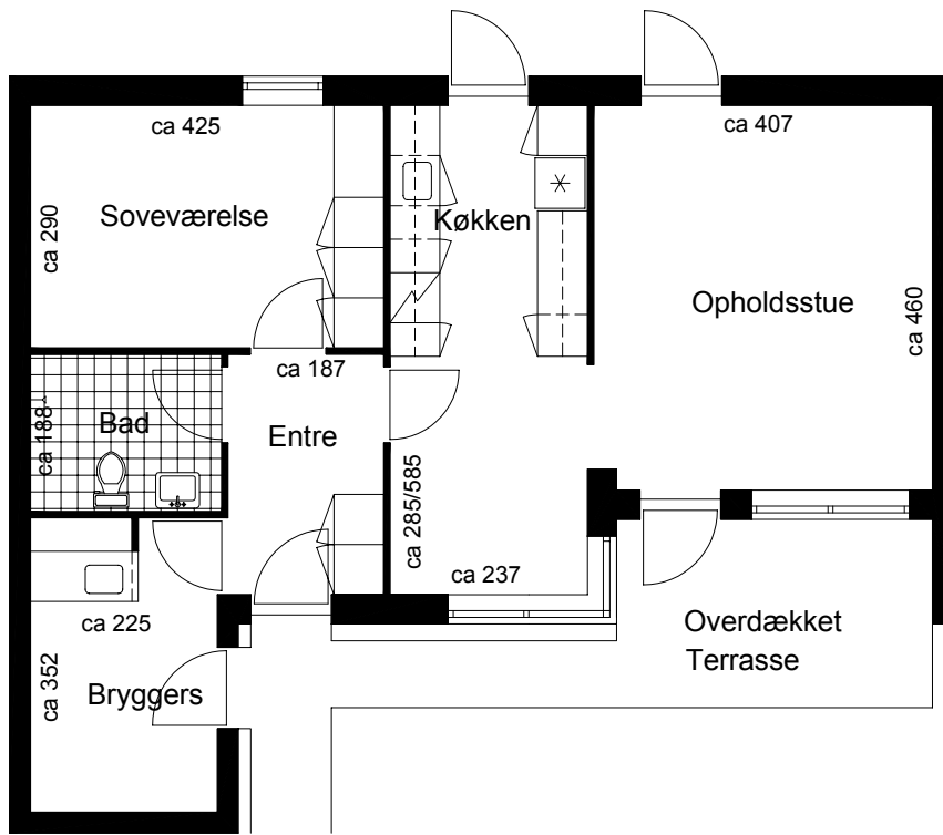
Plantegning
