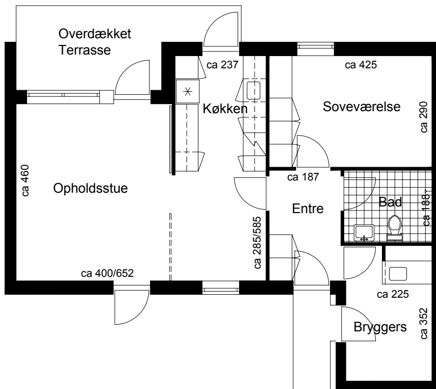
Plantegning
