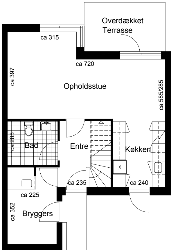
Stueplan
