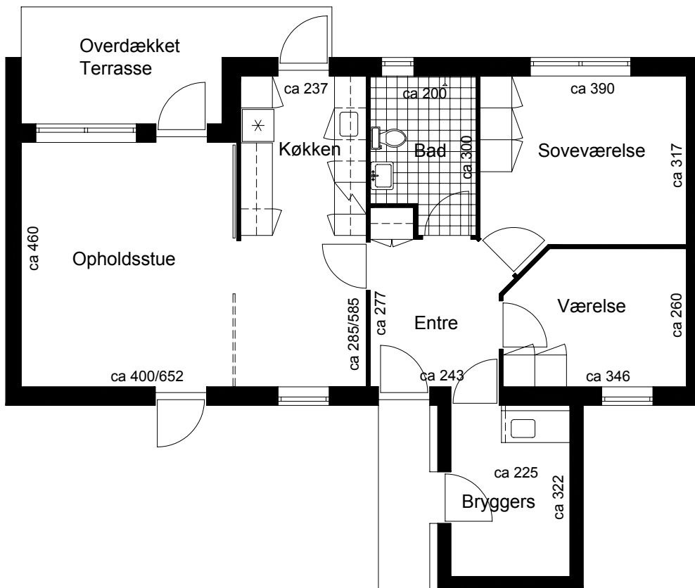
Plantegning
