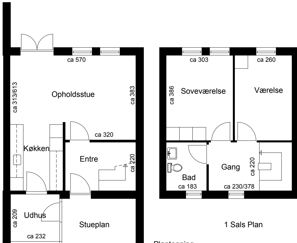
Plantegning
