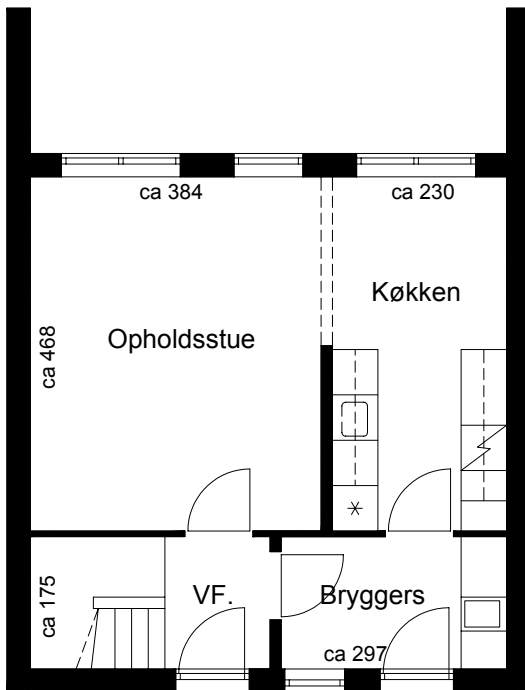
Stueplan
