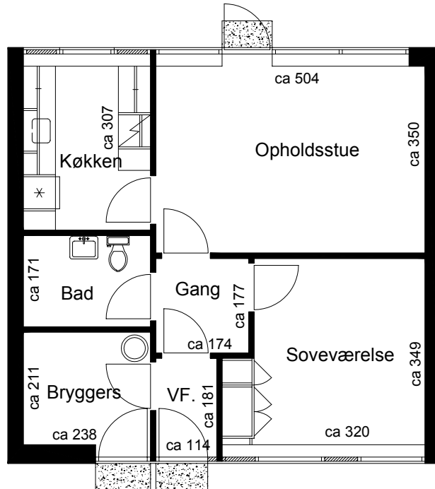
Plantegning
