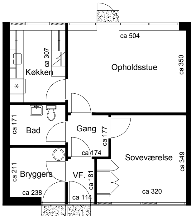
Plantegning
