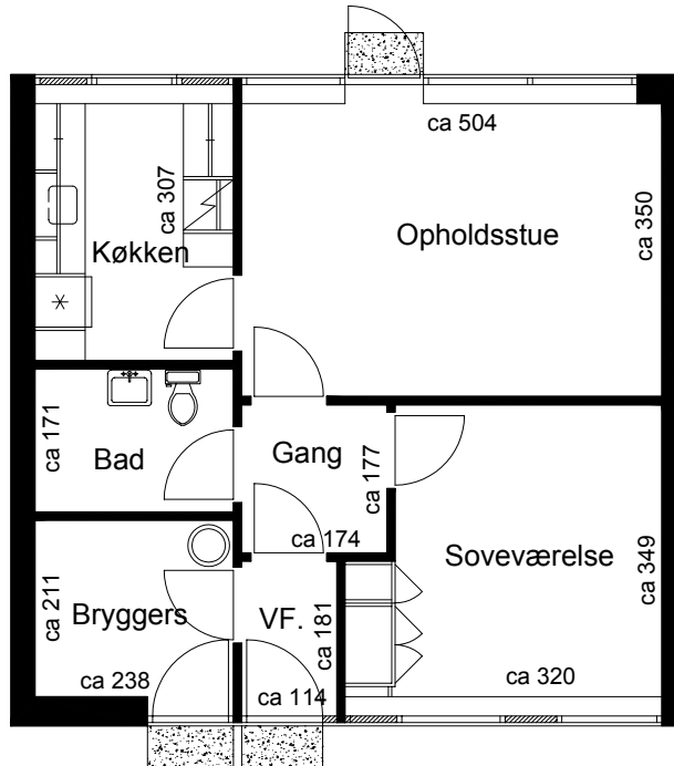
Plantegning
