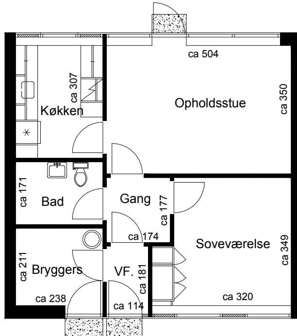
Plantegning
