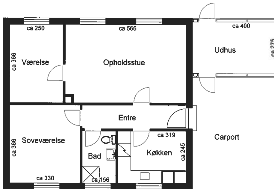
Plantegning
