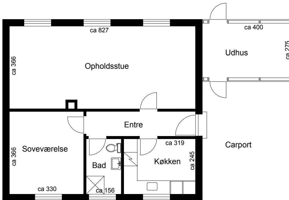
Plantegning
