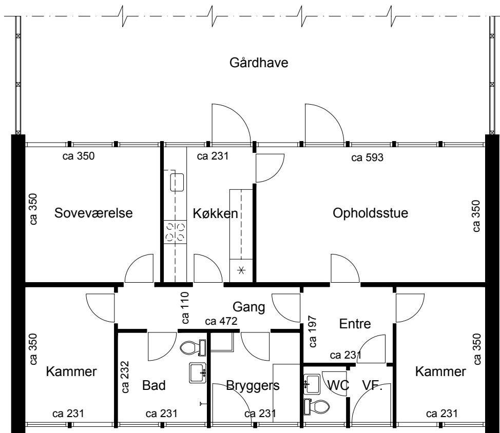
Plantegning
