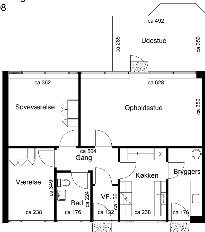
Plantegning
