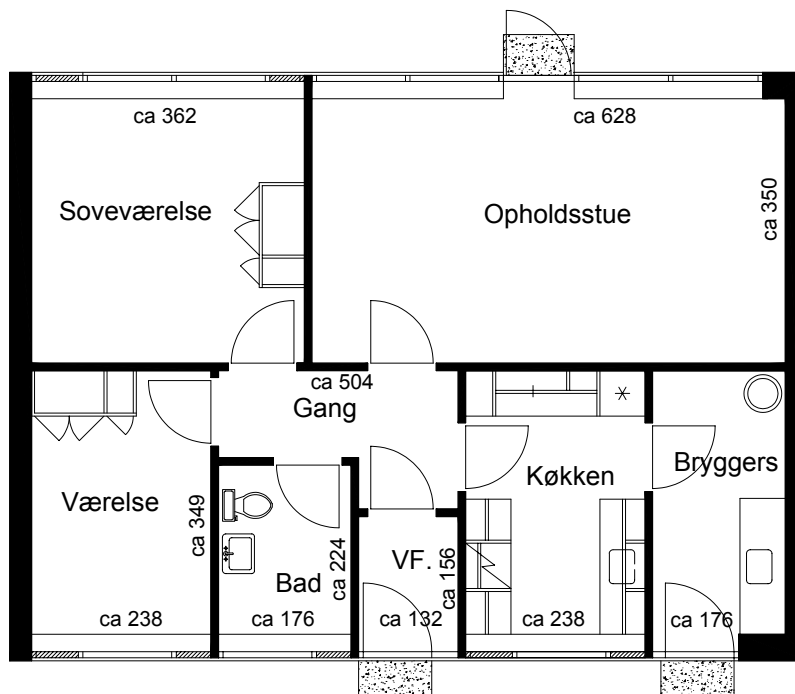
Plantegning
