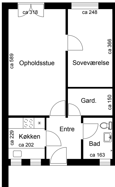
Plantegning
