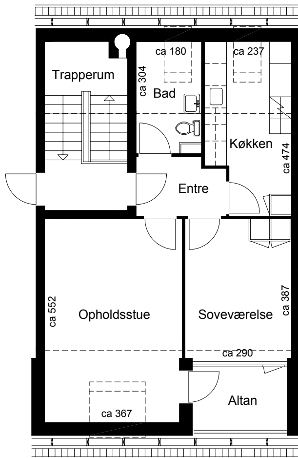
Plantegning
