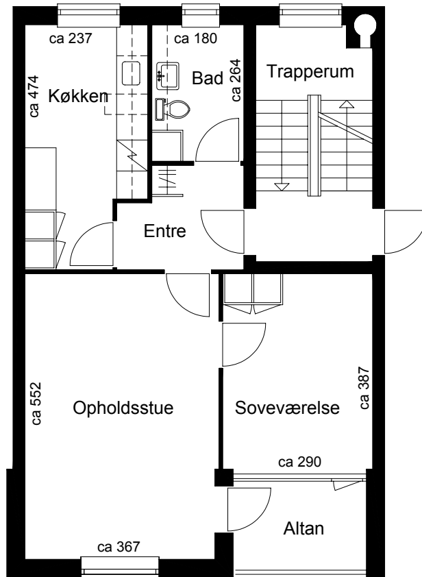
Plantegning
