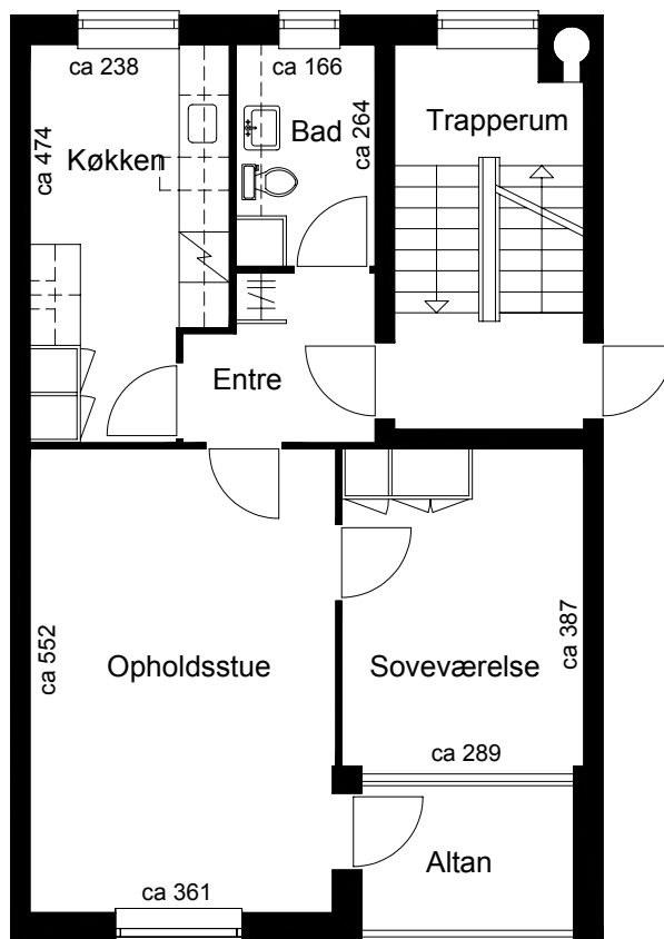
Plantegning
