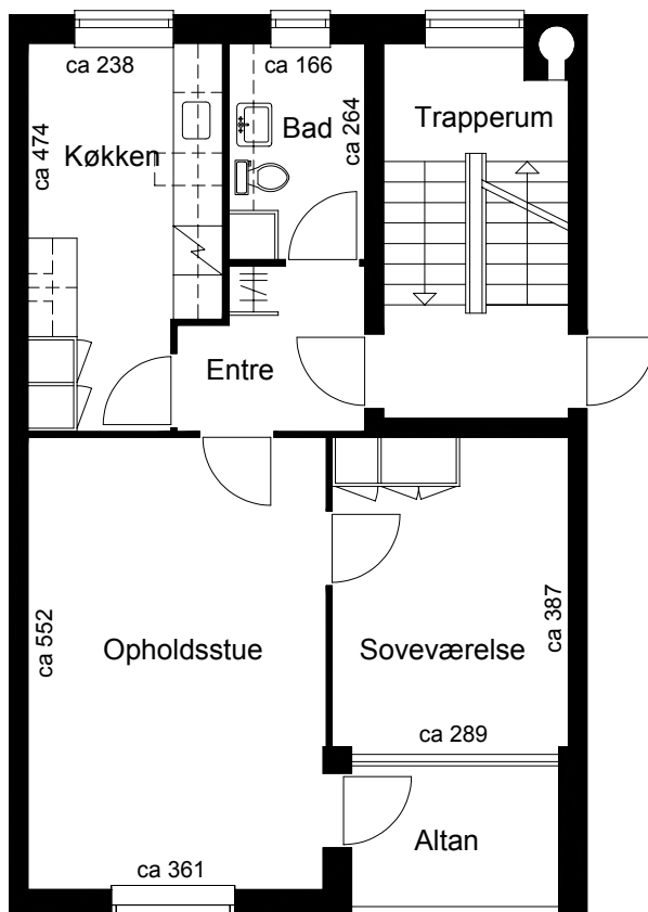
Plantegning
