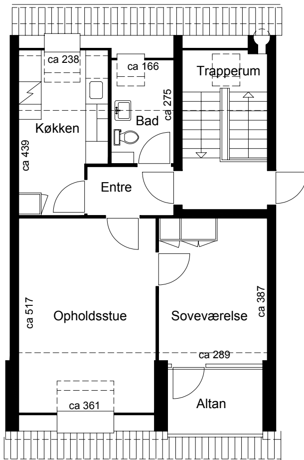
Plantegning
