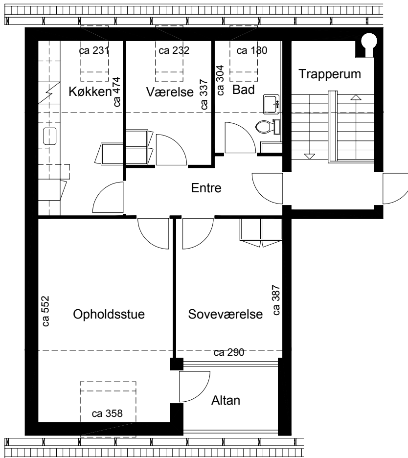
Plantegning
