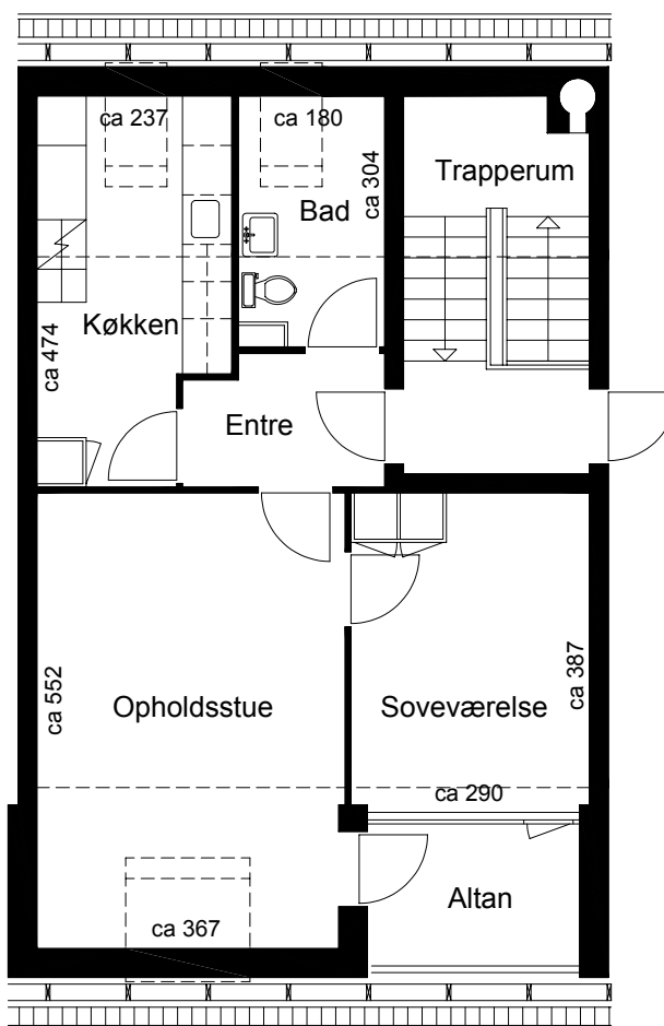
Plantegning
