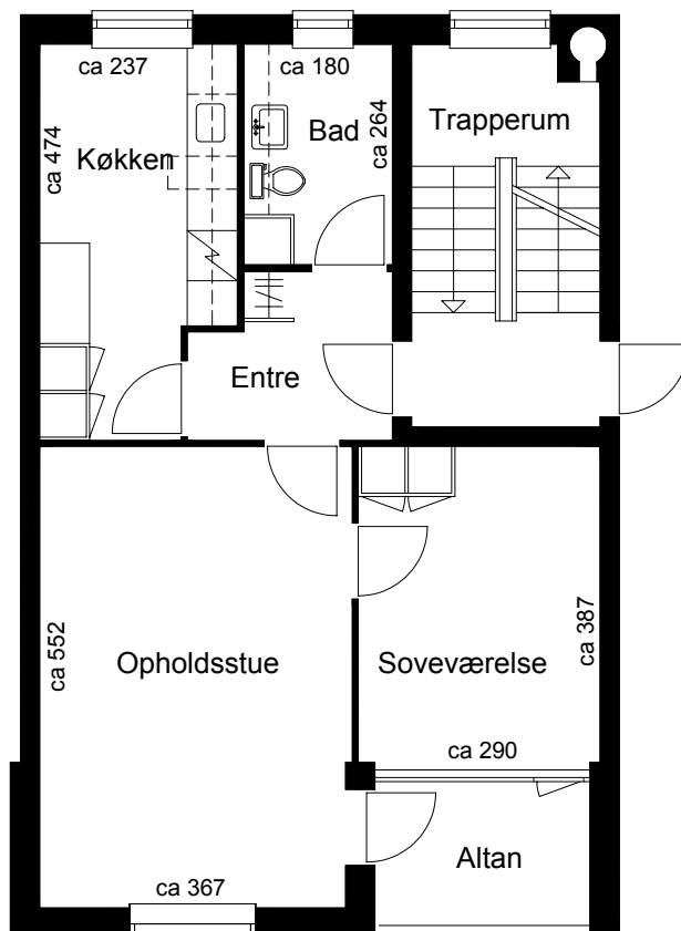
Plantegning
